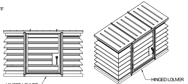
HINGED DOOR
